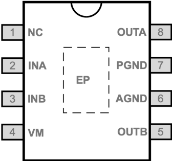
图2. LTK8530管脚说明
